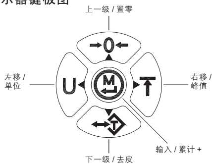
称重显示器键板图
